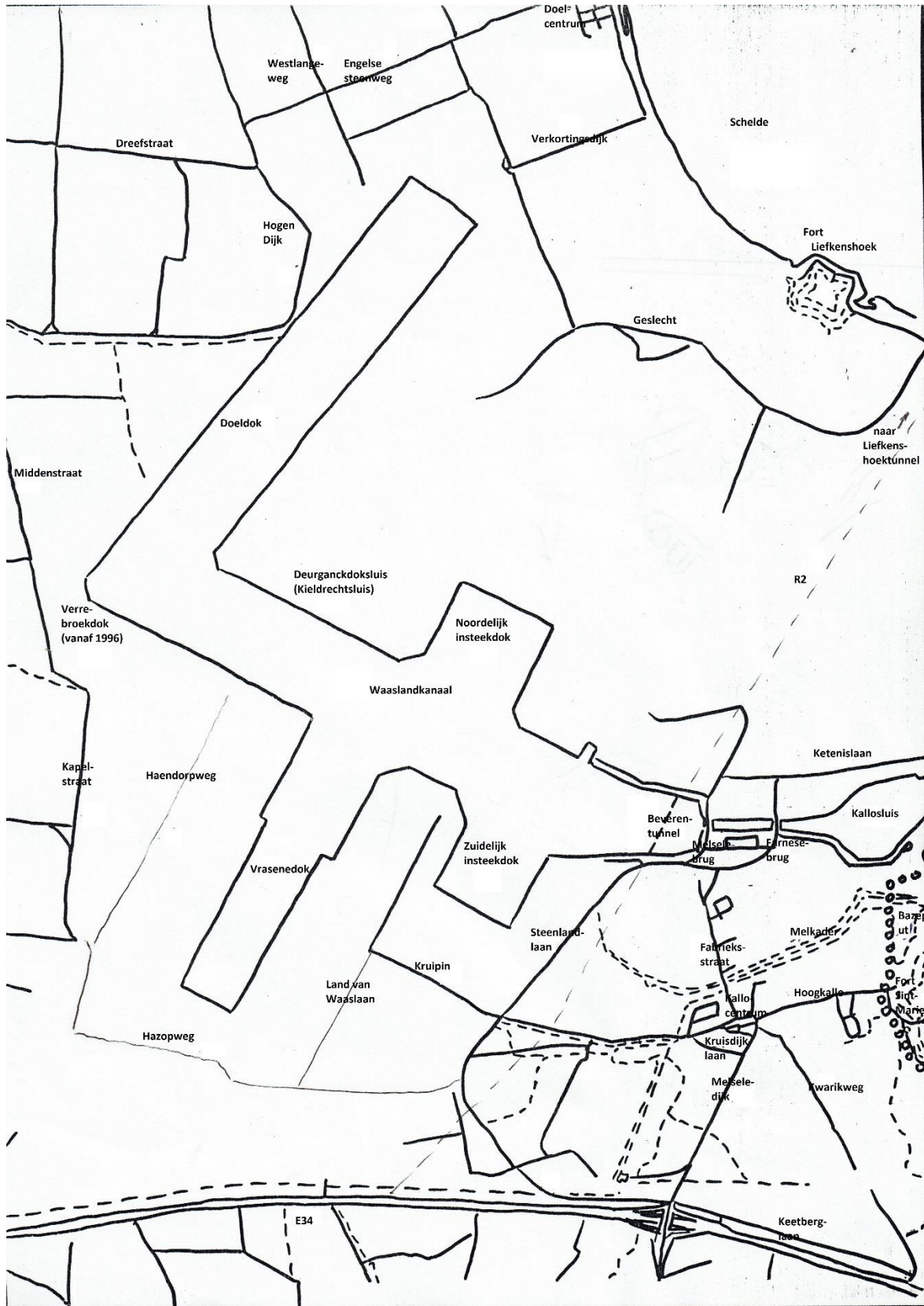
Kaartje Waaslandhaven (eigen collectie, 1985). Het Deurganckdok ligt ongeveer evenwijdig aan en onder het Doeldok. De Deurganckdoksluis –nu Kieldrechtsluis– maakt de verbinding met het Waaslandkanaal.
